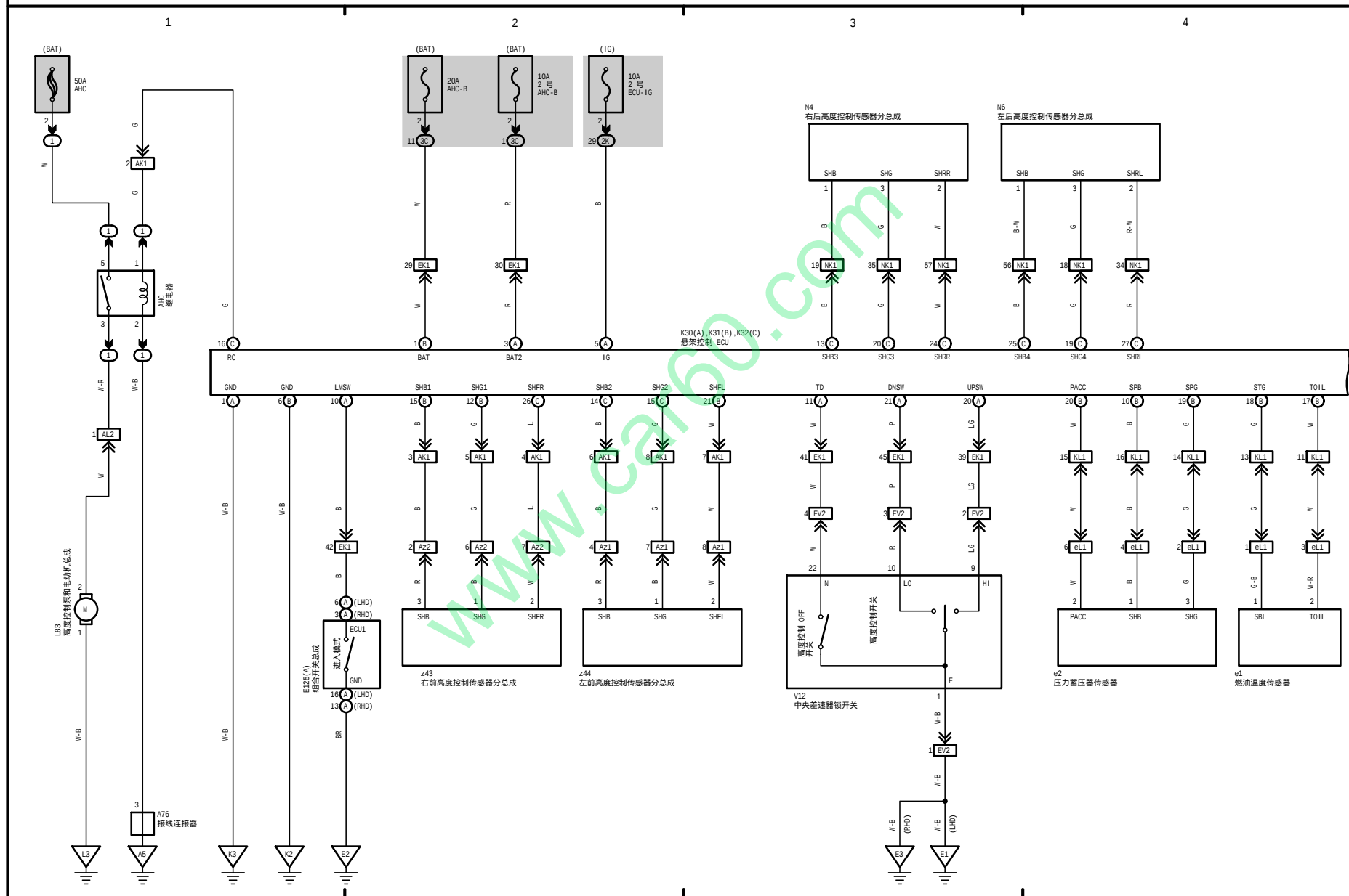
主动高度控制悬架和自适应可调悬架 (2015 年 9 月之后生产)
